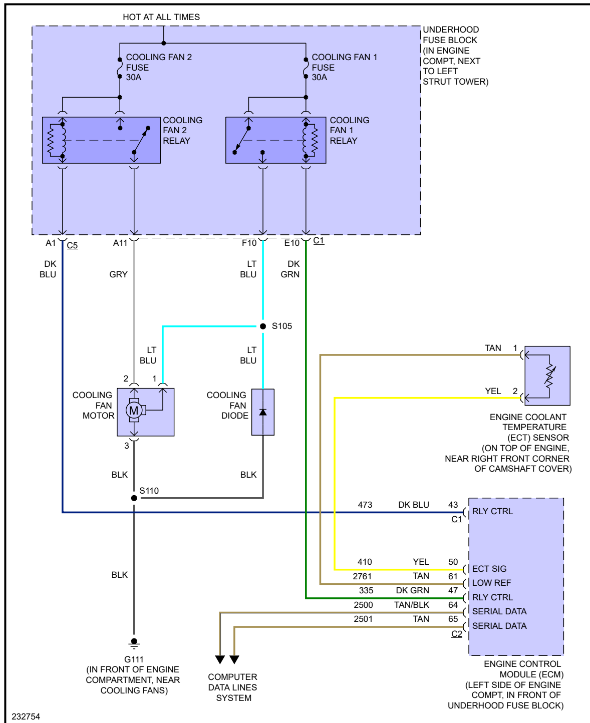
Fig 1: 2.2L VIN F, Cooling Fan Circuit
