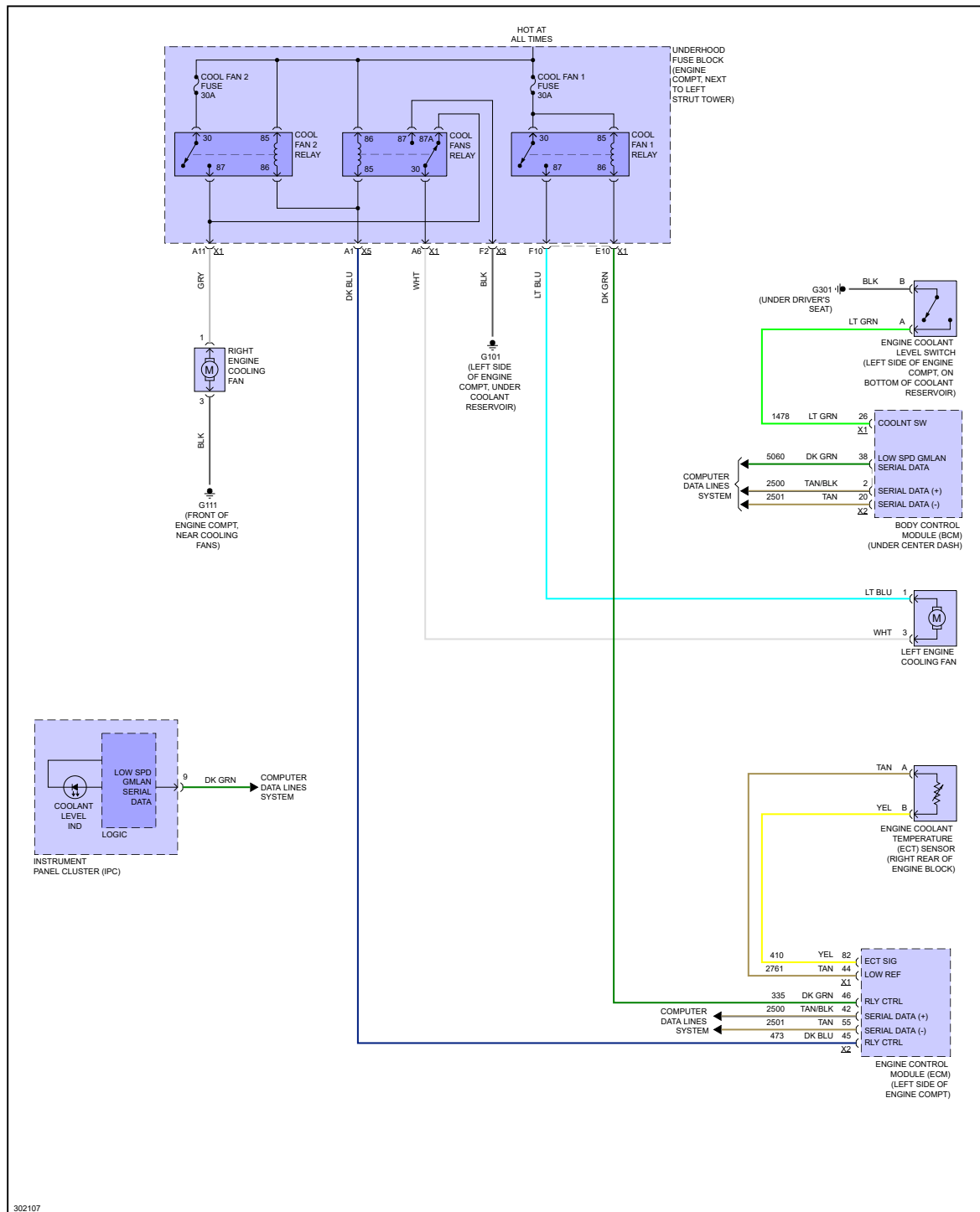
Fig 1: 2.0L VIN X, Cooling Fan Circuit
