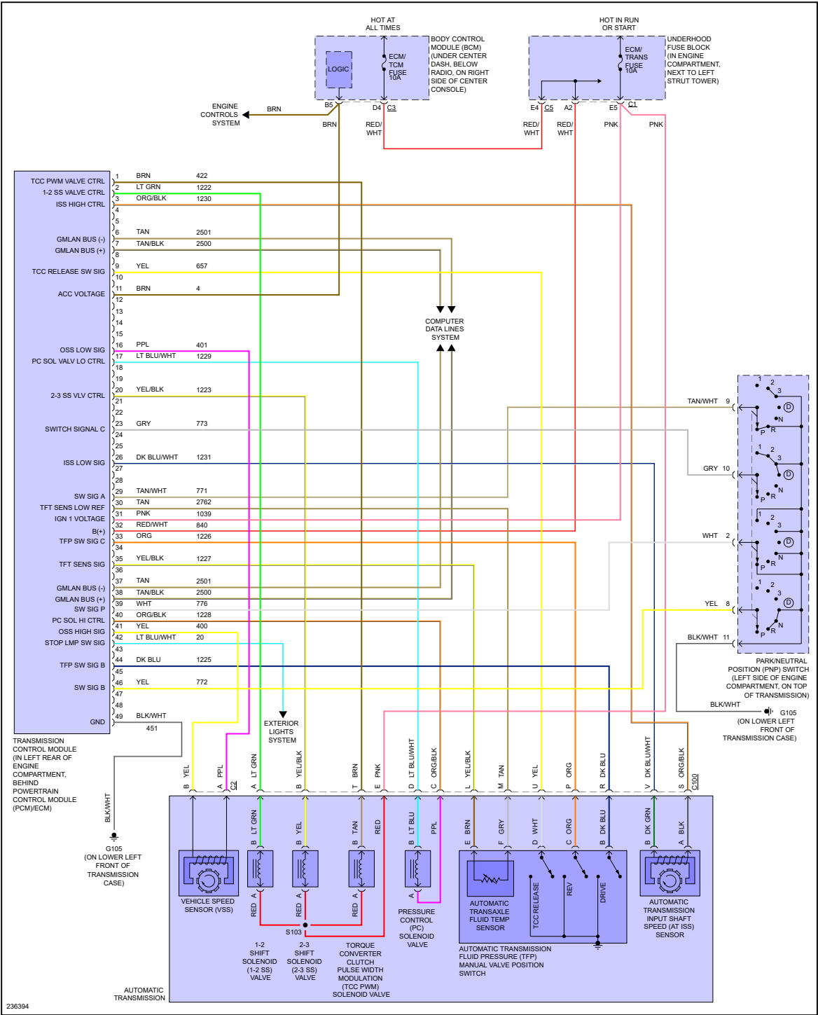
Fig 1: 2.4L VIN B, A/T Circuit
